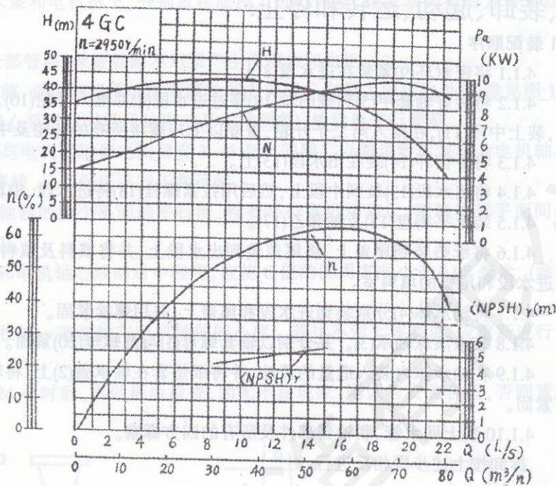
4GC-8 型离心水泵性能表
