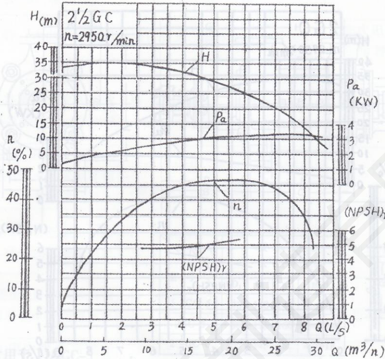
2 1/2 GC-6 型离心水泵性能表
