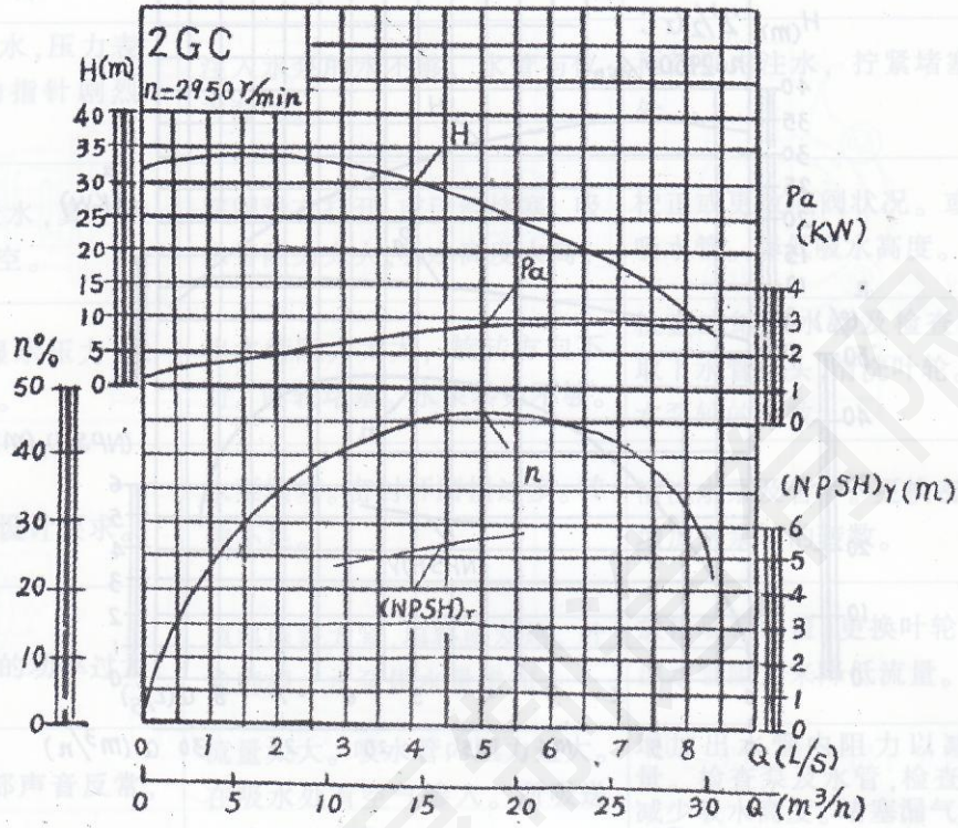
2GC-5 型离心水泵性能表
