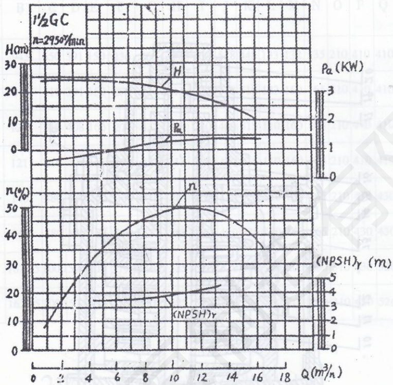
1 1/2GC 型离心水泵性能曲线图
